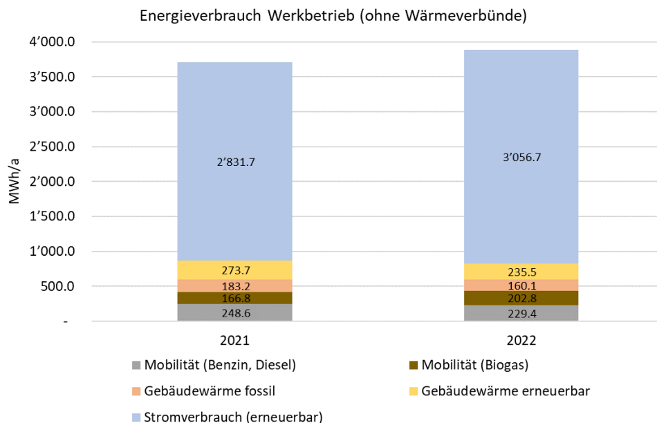
Abbildung 9: Energieverbrauch innerhalb der Organisation (ohne Wärmeverbände)
