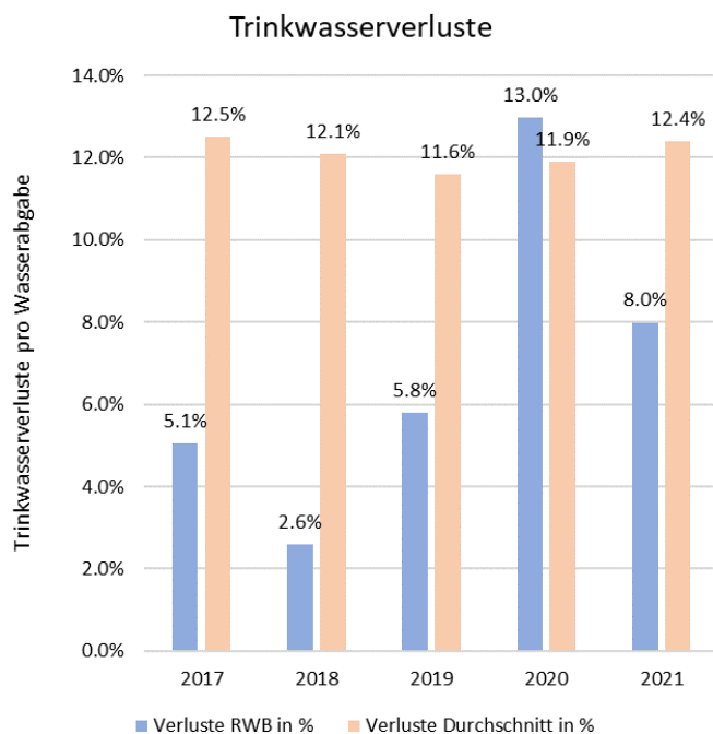
Abbildung 4: Trinkwasserverluste
