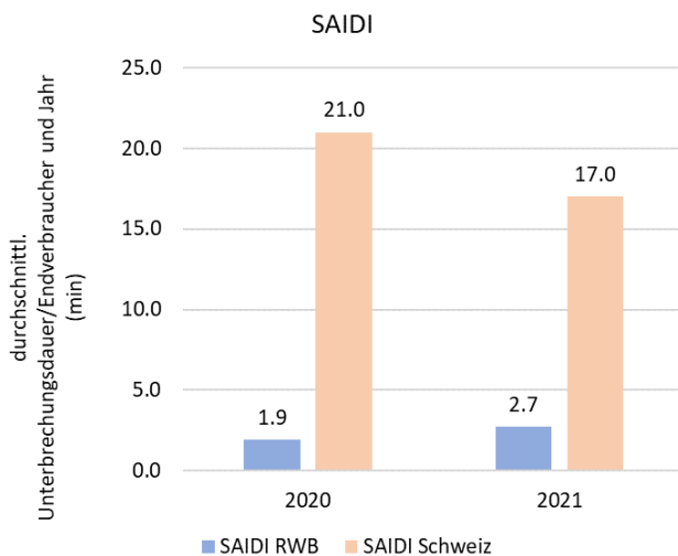
Abbildung 3: SAIDI
