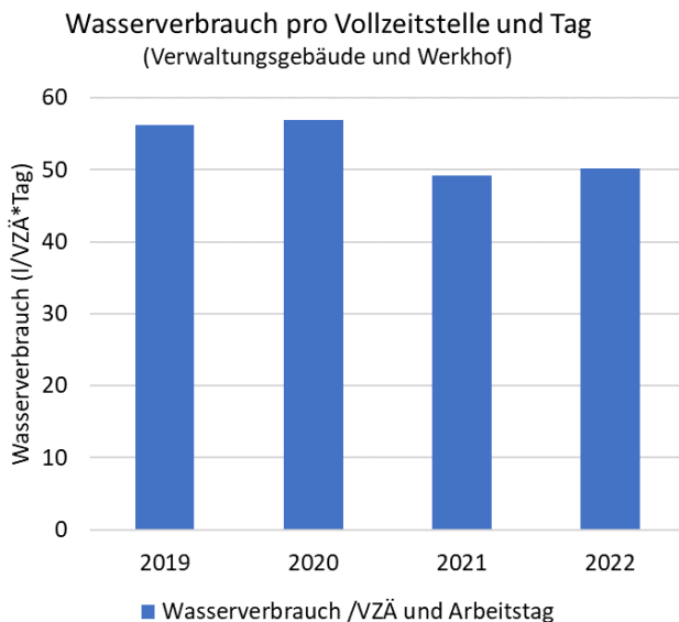
Abbildung 20: Wasserverbrauch (Verwaltung und Werkhof) pro Mitarbeiter/in (Vollzeitäquivalente)
