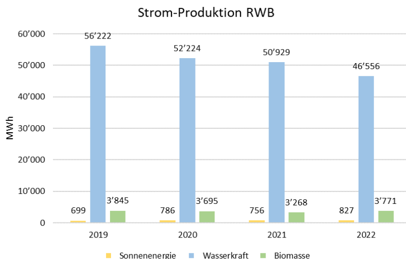
Abbildung 14: Stromproduktion
